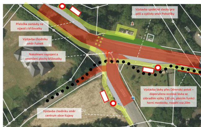
IDEOVÝ NÁVRH ÚPRAV KŘÍŽOVATKY A ZASTÁVEK NA SILII/647 V OBCI KUJAVY - CÍLOVÉ ŘEŠENÍ VARIANTA A - SITUOVÁNÍ ZASTÁVEK NA VÝJEZDU Z KŘÍŽOVATKY SE SPOLEČNÝM ODBAVENÍM VŠECH SPOJŮ SMĚRUJÍCÍCH DO DANÉHO SMĚRU
