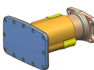
Nárazník s plastovou deskou, šířka talíře 550 mm
