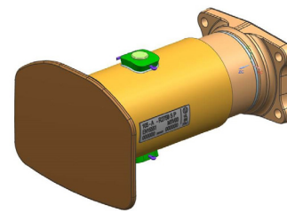
Nárazník nové konstrukce s nižšími výrobními náklady (v modelu talíř šířky 450 mm)
