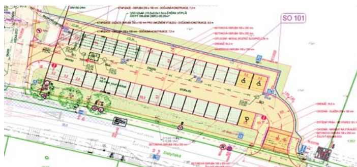
Koordinační situační výkres 1. etapy.
