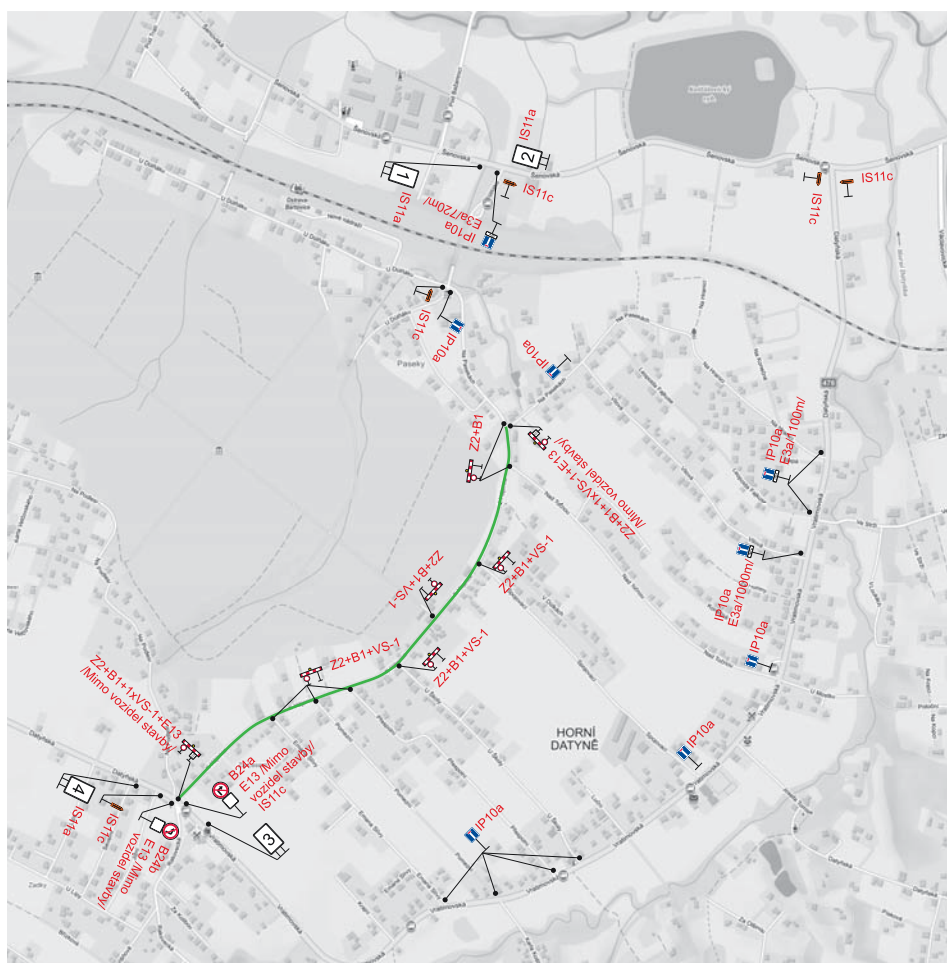
Situční výkres uzavírky
