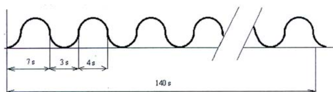
Obrázek č. 2. - Schéma průběhu signálu Všeobecná výstraha (ES)
