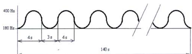
Obrázek č. 2. - Schéma průběhu signálu Všeobecná výstraha (ES)
