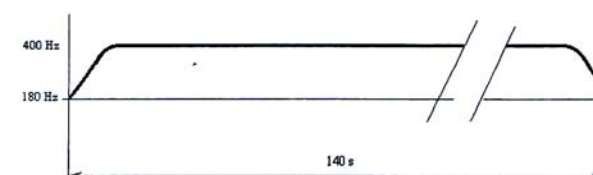
Obrázek č. 6. - Schéma průběhu Zkušební tónu (ES)
