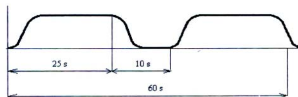
Obrázek č. 4. - Schéma průběhu signálu Požární poplach (ES)
