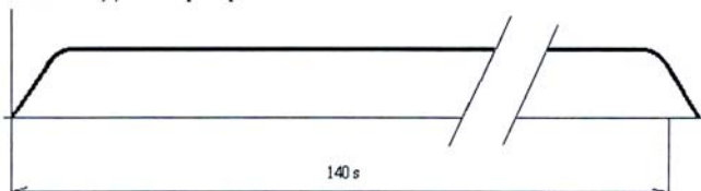
Obrázek č. 6. - Schéma průběhu Zkušební tónu (ES)
