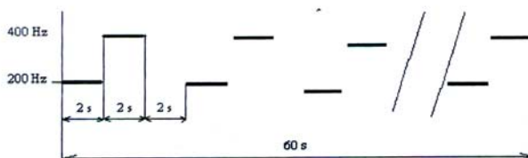
Obrázek č. 4. - Schéma průběhu signálu Požární poplach (ES)
