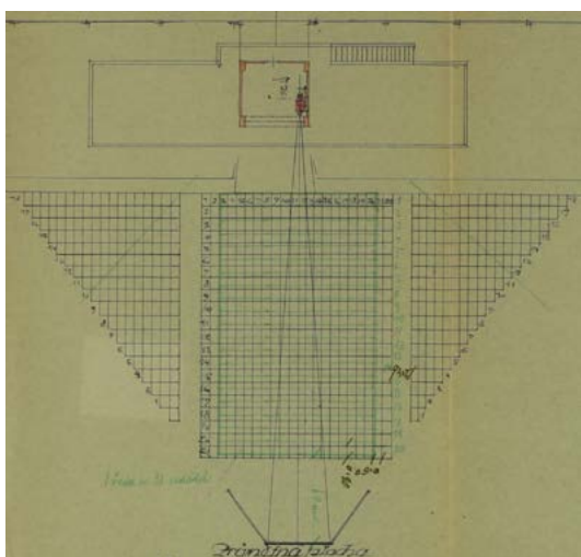
Projekční návrh areálu letního kina situovaného na cvičišti Sokola se zakresleným hledištěm a pavilonem, ve kterém měl být instalován promítací stroj. Repro | Státní okresní archiv Karviná
