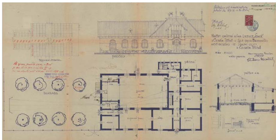
Projekční návrh úprav společenského sálu pro účely kina Sport v restauraci Aloise Branného. Repro | Státní okresní archiv Karviná
