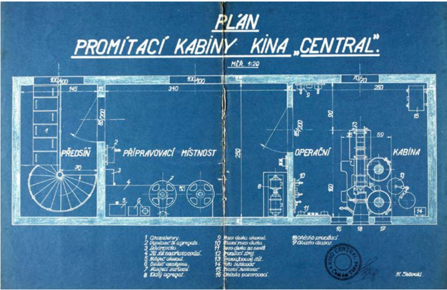
Uspořádání promítací kabiny dle návrhu architekta Karla Gottwalda. Repro | Státní okresní archiv Karviná
