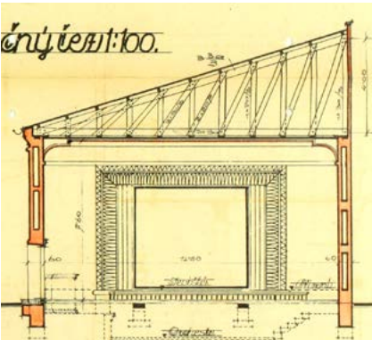
Výřez z projektové dokumentace - příčný řez s pohledem na jeviště a orchestríště. Repro | Státní okresní archiv Karviná
