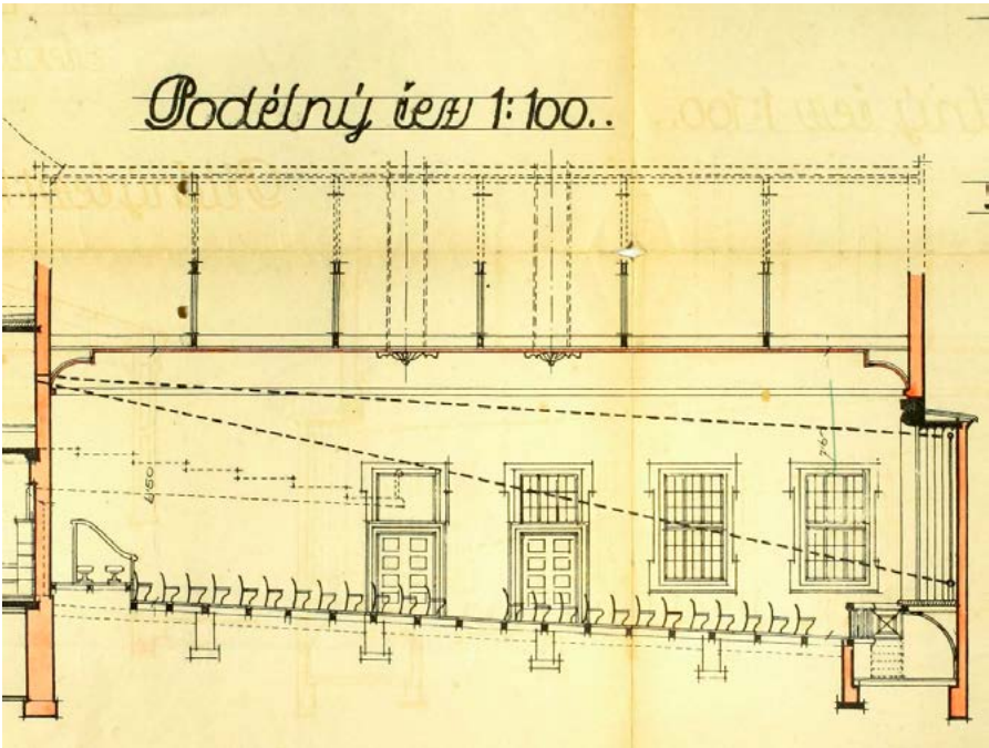
Výřez z projektové dokumentace - podélný řez hledištěm. Repro | Státní okresní archiv Karviná
