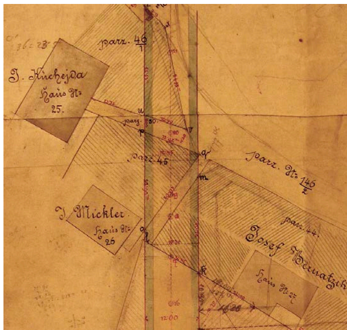
Situační plán z roku 1881 zobrazuje vytyčení budoucí Hasnerovy ulice (nyní Sokola-Tůmy). V jejím okolí je vidět dnes již neexistující roztroušená zástavba. Zleva: Kucheidův dům č. 25, Miklerův dům č. 26, Bernatzkův dům č. 27.
