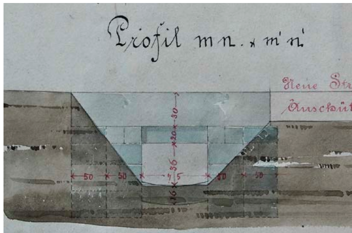
Příčný řez kamenným můstkem, jehož cílem bylo překlenutí vodního příkopu.
