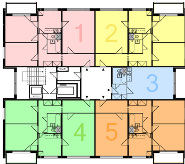
Půdorys podlaží.
