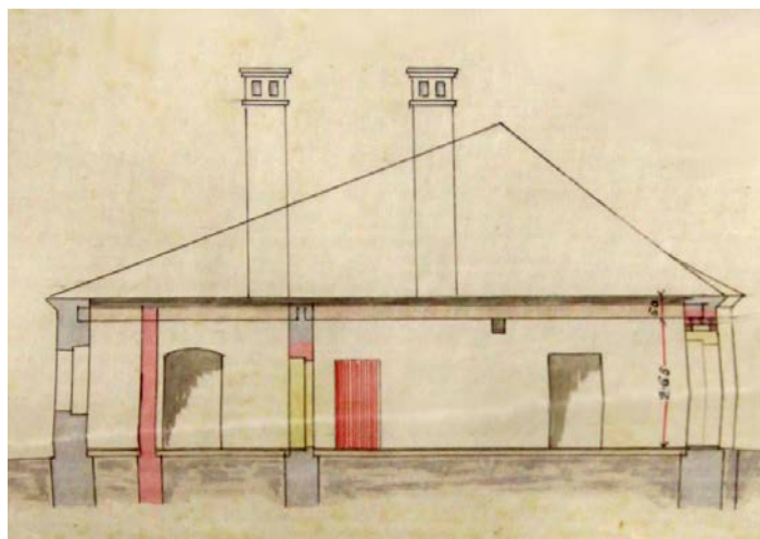
Příčný řez domem Franze Frisy, který měl být postaven v roce 1808 a zbourán v 1897.
