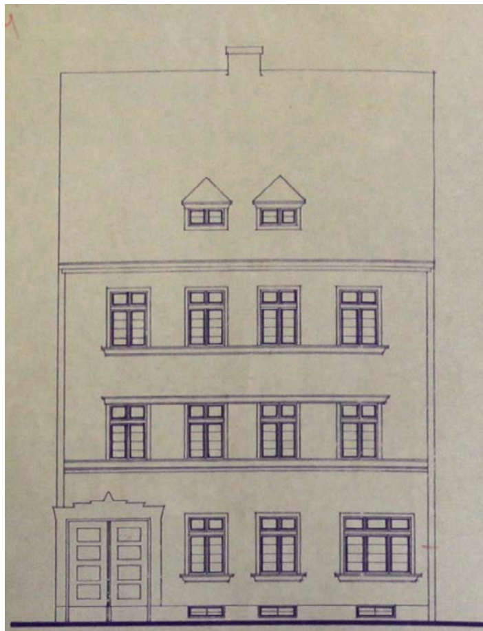
Čelní fasáda domu Rudolfa Maliny. Výřez z projektové dokumentace z roku 1931.
