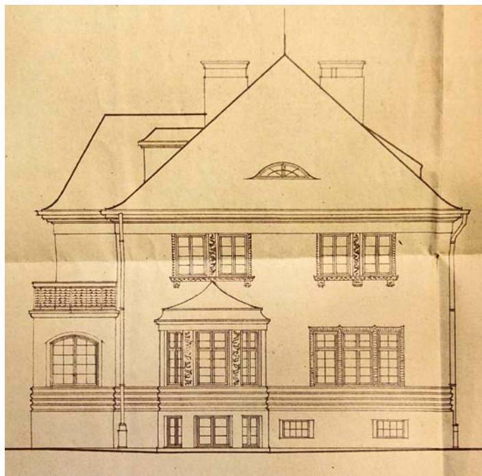
Výřez z projektové dokumentace znázorňuje pohled na fasádu vily Rudolfa Peschky z Illichovy třídy (ul. Moskevská). REPRO | STAVEBNÍ ARCHIV MĚSTA ČESKÝ TĚŠÍN
