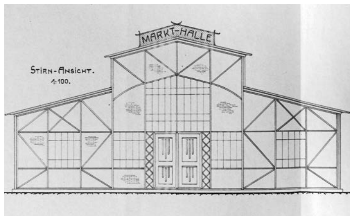
Čelní stěna haly dle návrhu Karlovy hutě v Lískovci.
