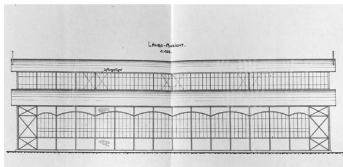
Bokorys haly dle návrhu Karlovy hutě v Lískovci.
