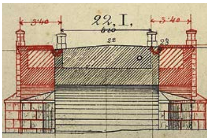
Příčný řez mostem navrženým městským inženýrem Kühnlem v roce 1883. Červená barva znázorňuje úpravu mostu. REPRO | ARCHIWUM PAŃSTWOWE W KATOWICACH
