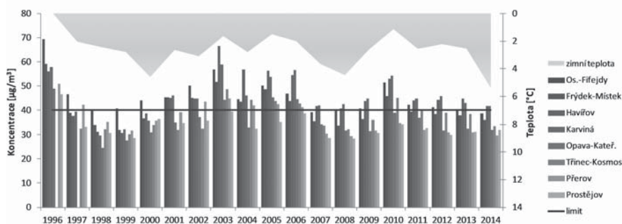
Obr. 11 - Roční průměrné koncentrace suspendovaných částic PM 10
