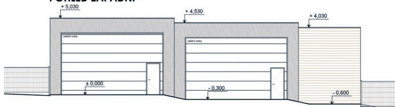
Výstavba nových garáží na ulici Černá cesta pro obecní techniku
