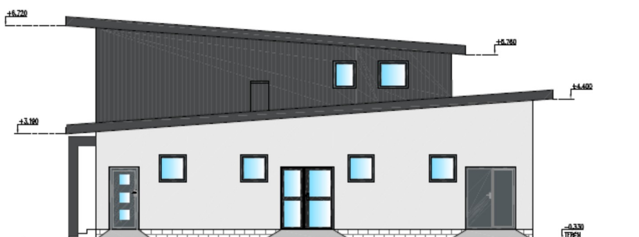
POHLED JIŽNÍ
