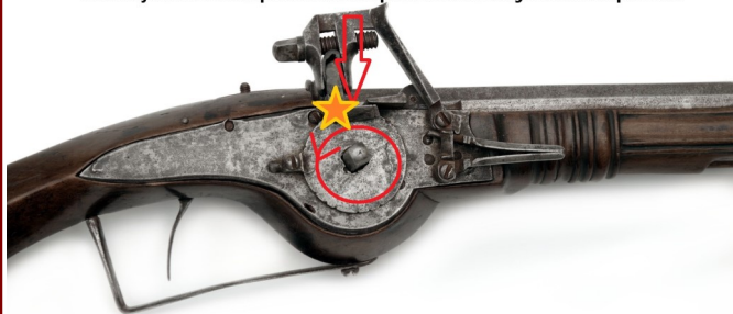
Kolečkový zámek. Obsluha pomocí natáhnutí péra a uvolnění energie křesadla na pánevku.
