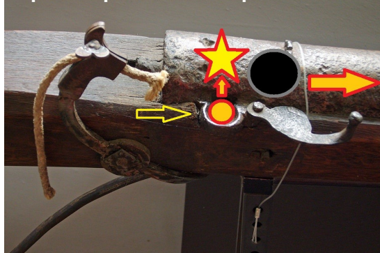
Doutnákový zámek princip přiložení doutnáku na pánevku s prachem následně odpálí slož v hlavní
