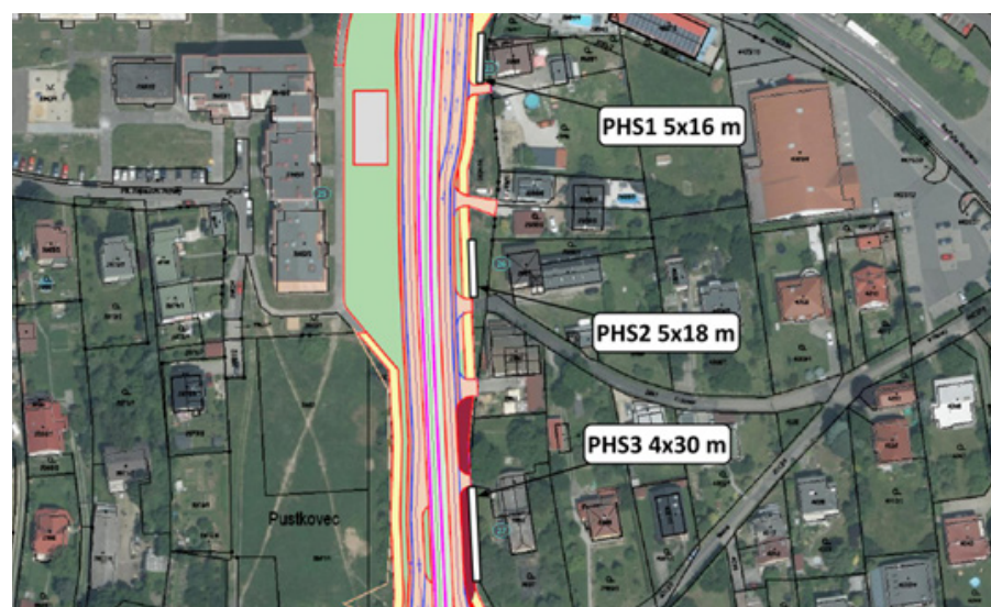
■ Umístění protihlukových stěn na ul. 17. listopadu v Pustkovci
