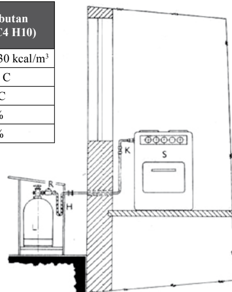
Obr. 1 Jednoduchá tlaková stanice na propan-butan
