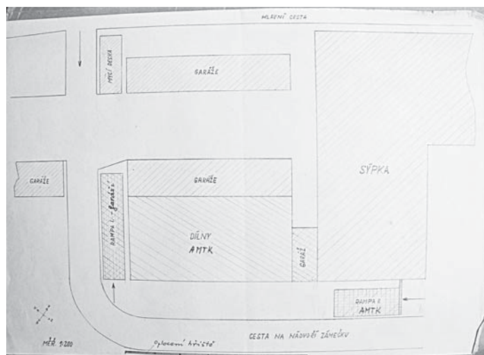
Plán rozmístění garáží
