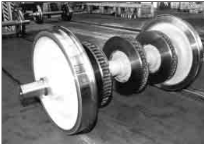
▲ Dvojkolí pro poschodové vozy rakouských drah
