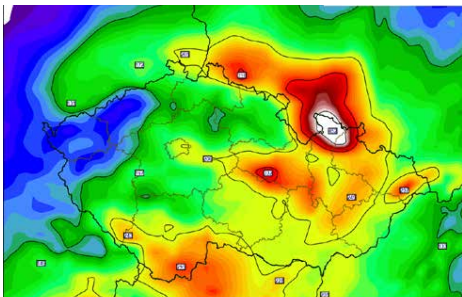
Matematický model úhrnu srážek za období od 11. 9. do 16. 9. 2024.
