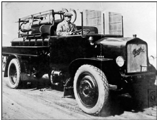
Hasicí vůz - výrobek továrny Oświęcim-Praga (vmax 5 km/h, spotřeba 15l / 100 km), www.ppoz.pl
