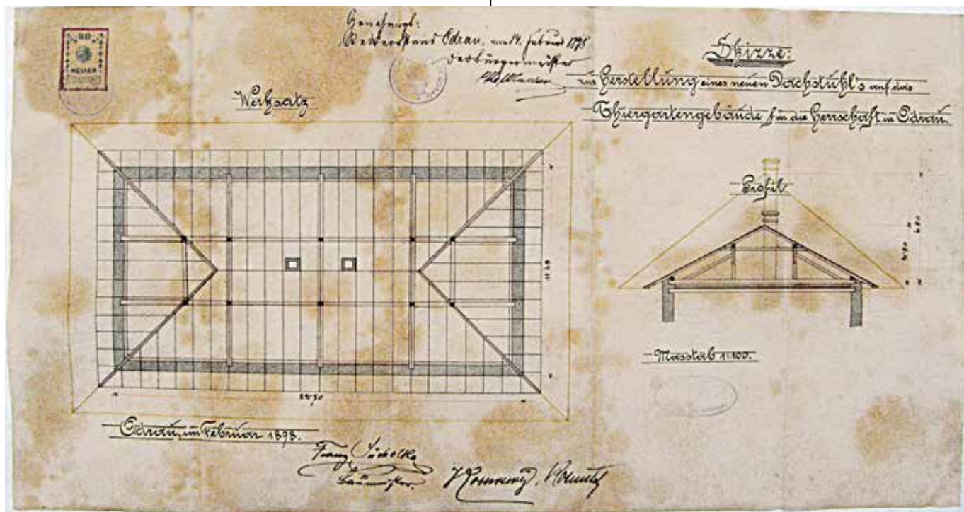
Návrh Franze Juchelky na nové zastřešení budovy hostince Tiergartenhaus, 1898. Archiv muzejního spolku Rolleder, o. p. s.
