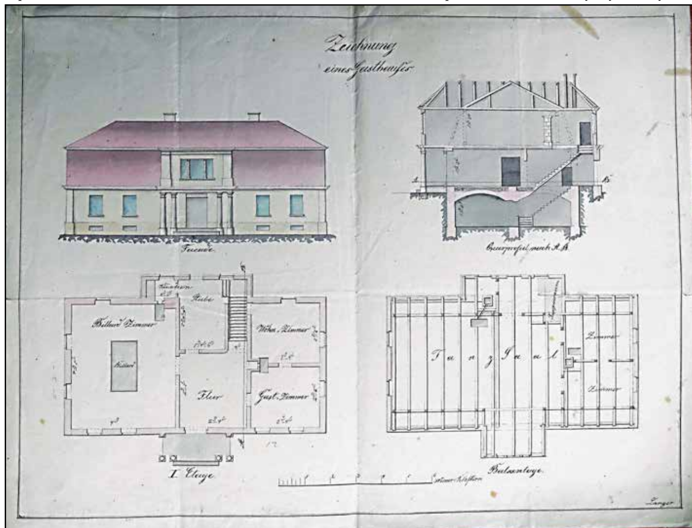
Langrův návrh I. přestavby hostince Tiergartenhaus. Archiv muzejního spolku Rolleder, o. p. s.
