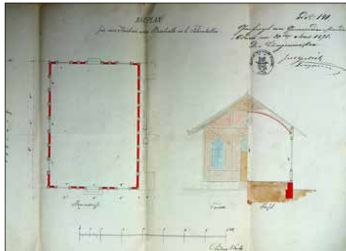
Stavební náčrt dřevěné tančírny stavitele Wankeho z roku 1871 pro II. Skalní sklep - panský hostinec. Archiv Emila Mateiciuca
