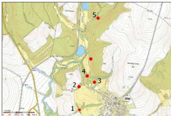
Viditelné terénní úpravy a stavby u Děrného: 1. Propustek přítoku Gručovky s náspem, 2. Terénní zářez pod Děrným, 3. Bývalá pískovna, 4. Nedokončený skalní zářez, 5. Propustek přítoku Gručovky u nedokončeného železničního mostu.
