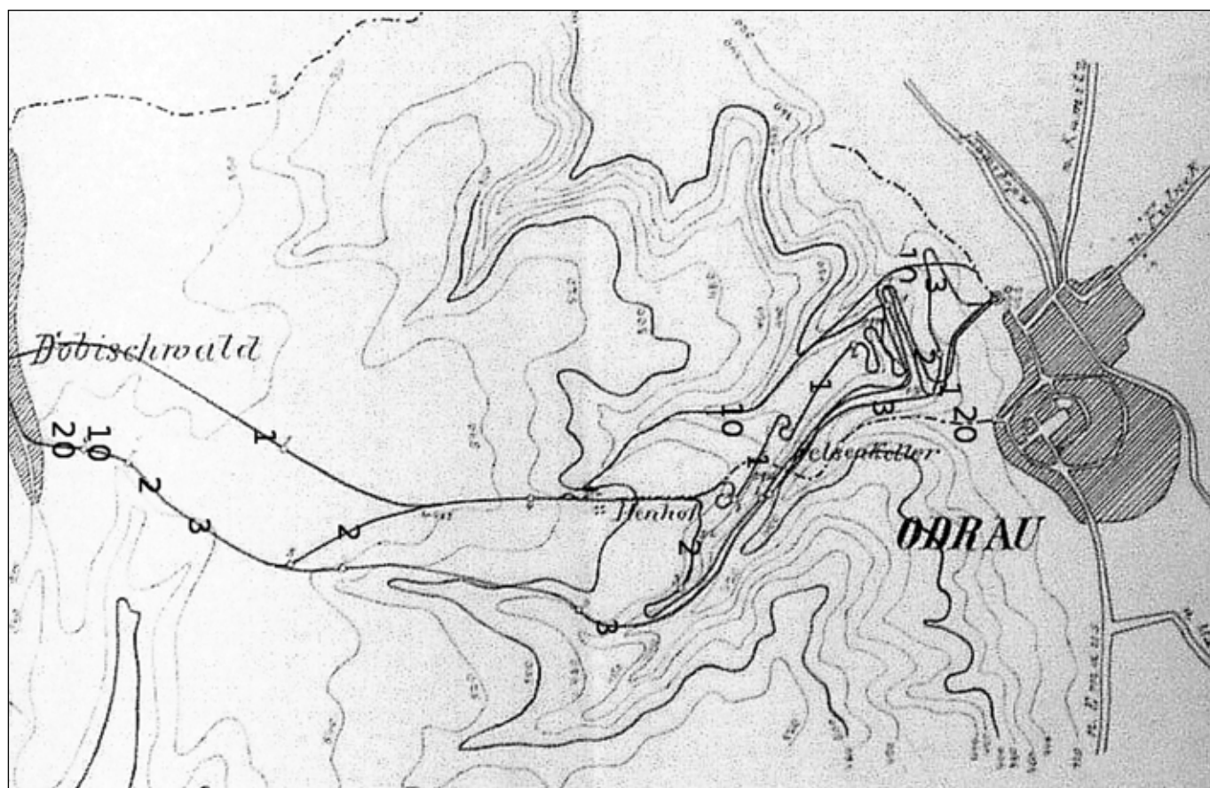
Tři varianty projektu (1, 2, 3) trasování horské silnice Odry – Dobešov. Zemský archiv Opava.
