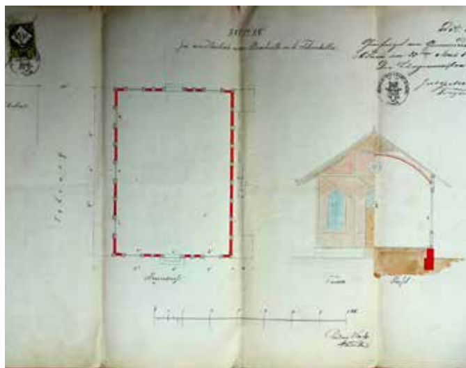
Stavební náčrt dřevěné tančírny stavitele Wankeho z r. 1871 pro II. Skalní sklep - panský hostinec
