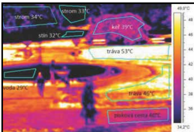
Pokosený trávník má teplotu 53°C, tráva 46°C, písková cesta 40°C, voda 29°C, stín pod stromy 32-34°C, keře 39°C
