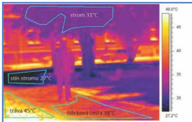
Teplota trávníku ve stínu stromu je 27°C, teplota trávníku na slunci je 45°C, teplota povrchu cesty 38°C a povrchu stromu 31°C
