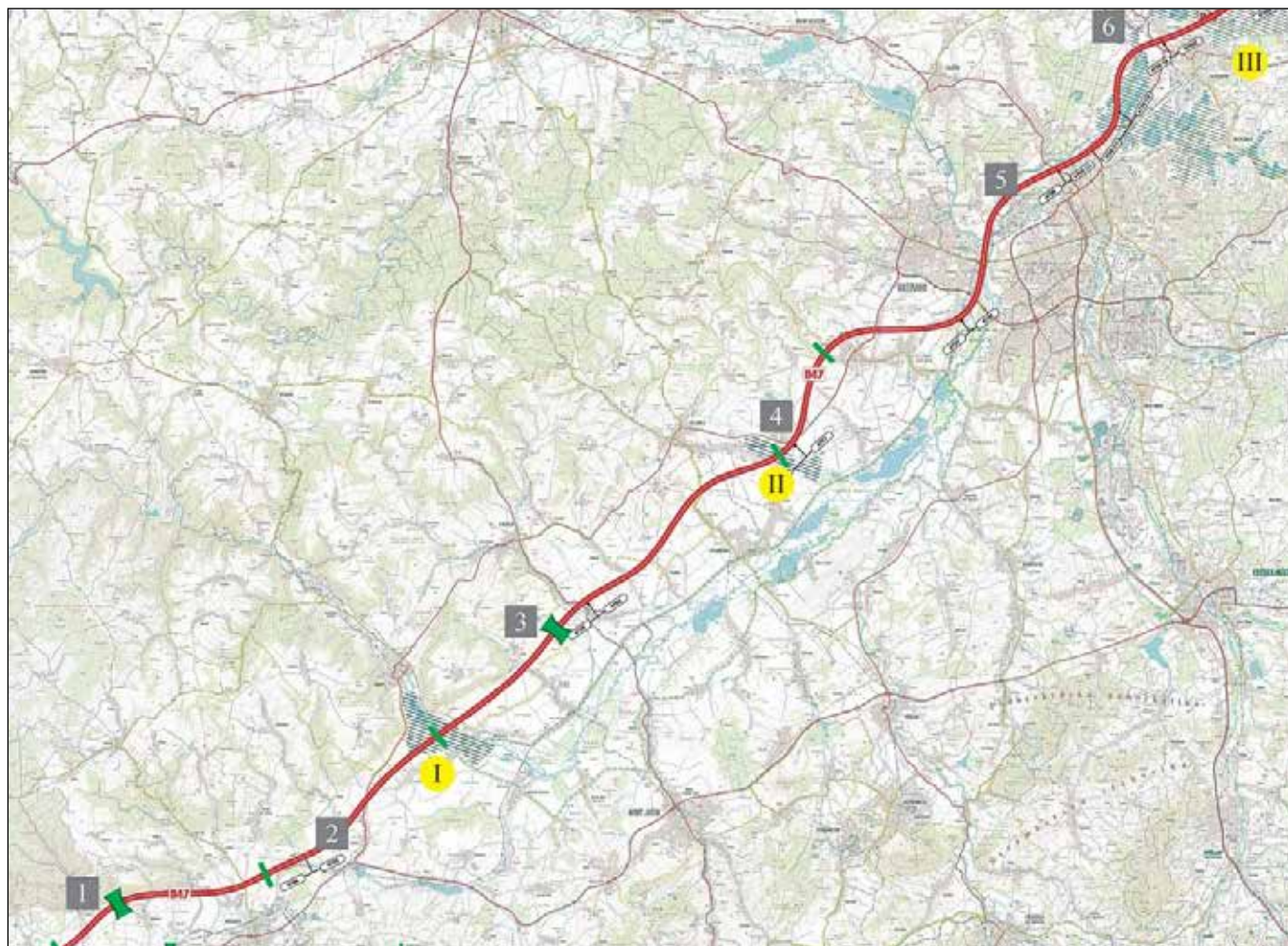
Řešení migračních tras velkých savců přes dálnici D47 na úseku 4705 - Bělátná - Hladké Životice. Zdroj: www.viamoravica.cz
