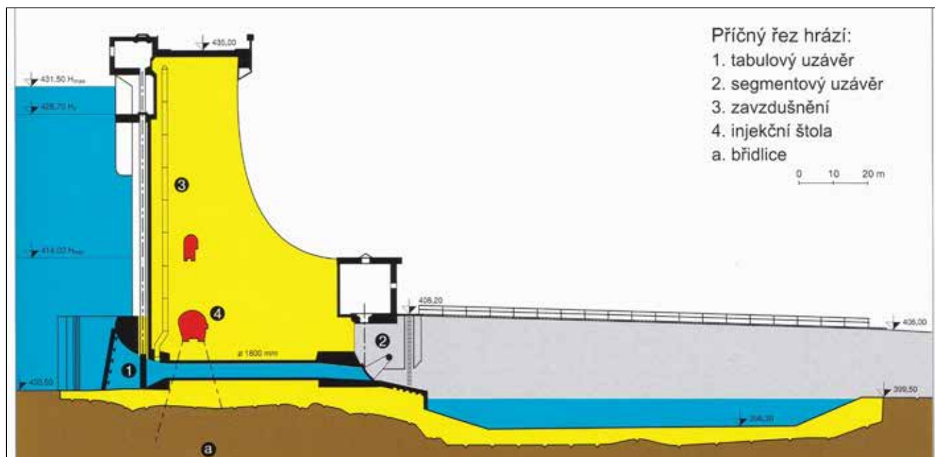
Schematický řez železobetonovým tělesem hráze se spodní výpustí, Zdroj: Kniha Povodí Odry Otty Brosche
