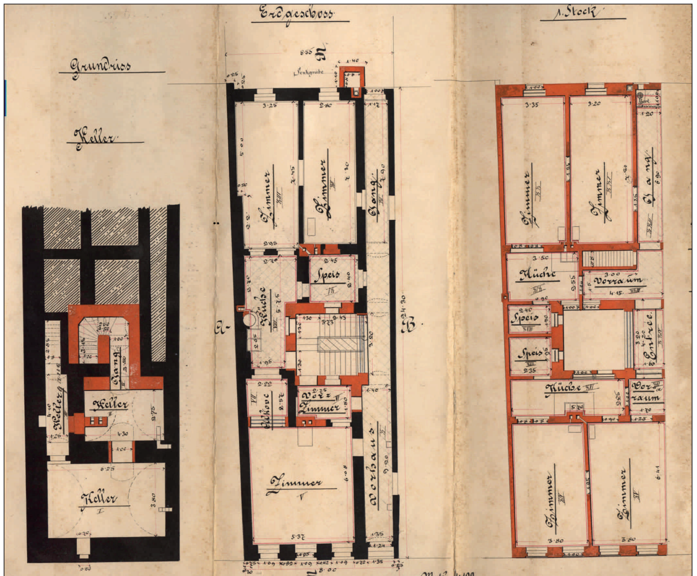
Stavební plány pro nadstavbu 2. patra pro dům Antona Rolledera na Hranické ulici v Odrách z roku 1886, půdorysy (autor stavebních plánů byl oderský stavitel Ludwig Wanke)
