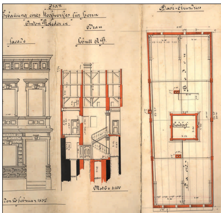
Stavební plány pro nadstavbu 2. patra pro dům Antona Rolledera na Hranické ulici v Odrách z roku 1886, řez a pohled na fasádu (autor stavebních plánů byl oderský stavitel Ludwig Wanke)
