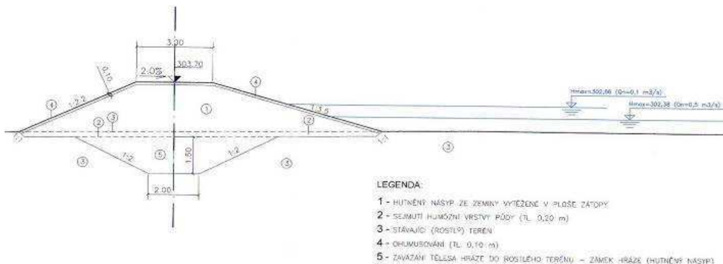
Vzorový příčný profil hráze (Atelier Fontes, s. r. o. Brno)
