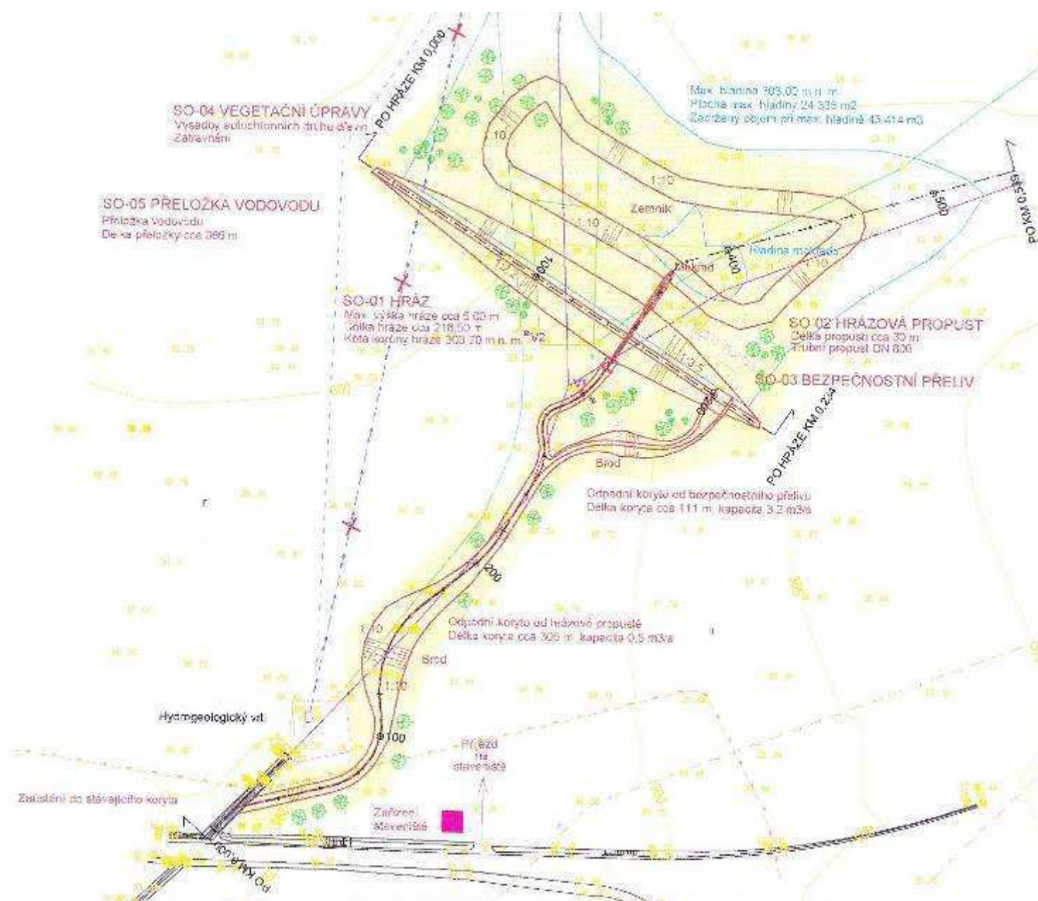
Podrobná situace stavby (Atelier Fontes, s. r. o. Brno)
