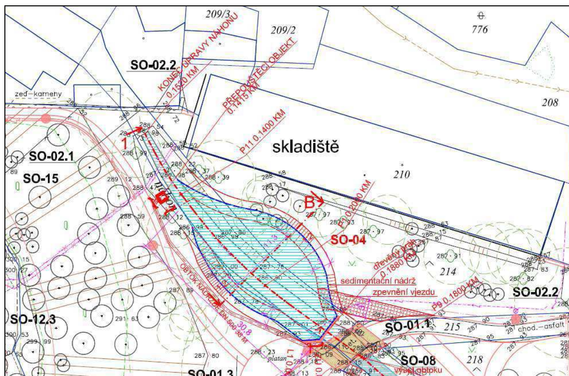
Sedimentační nádrž na náhonu u platanu (součást SO-04 Úprava náhonu)
