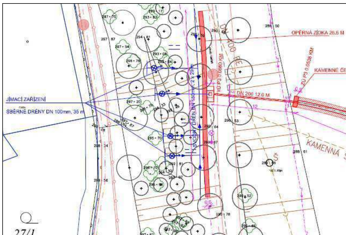
Úprava prameniště pod farou (SO-06)
