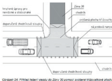
Obrázek 24. Příklad řešení vjezdu do Zóny 30 pomocí zvýšené křižovatkové plochy
