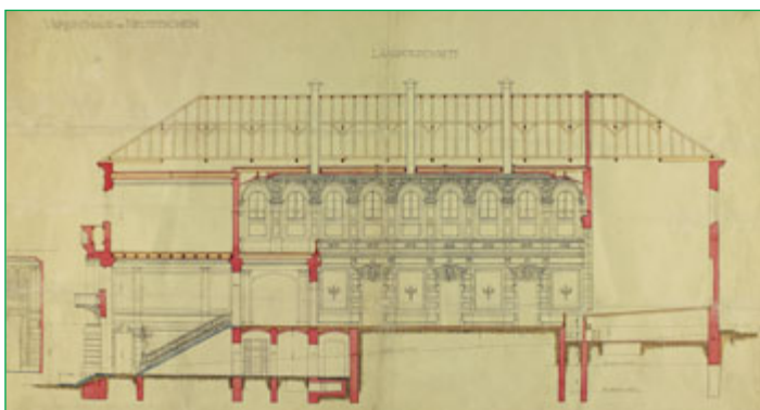
Plán stavby Německého spolkového domu z roku 1885
