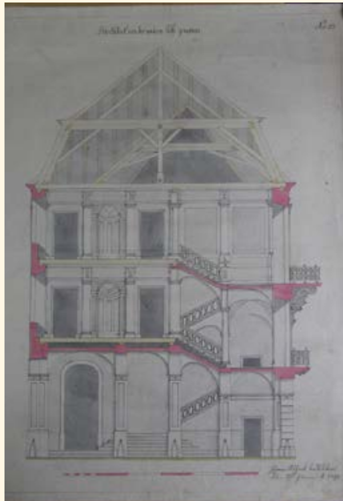
Johann Michael Badstüber, návrh úprav hlavního schodiště v zámku Bruntál, 1798.
