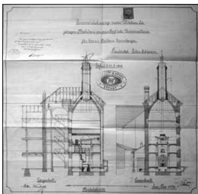
Projekt úpravy sladovny z konce 19. století.
