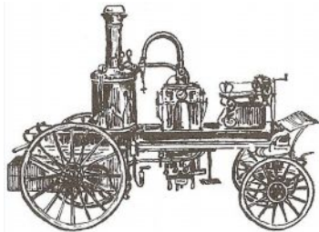
Parní stříkačka z roku 1884
