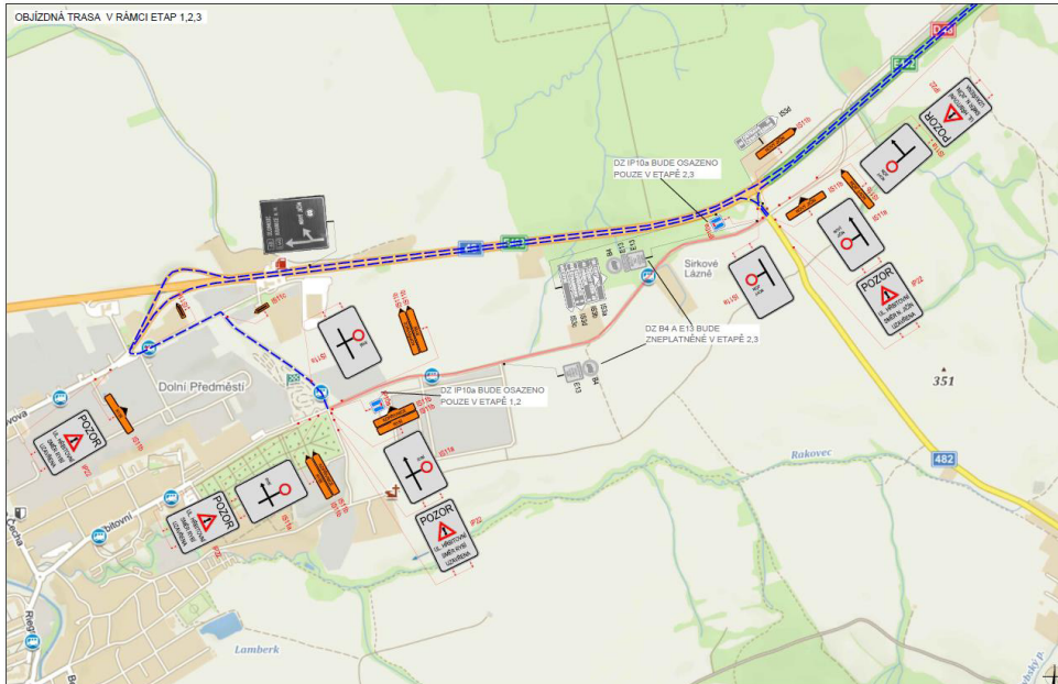
Situační výkres objízdné trasy.
