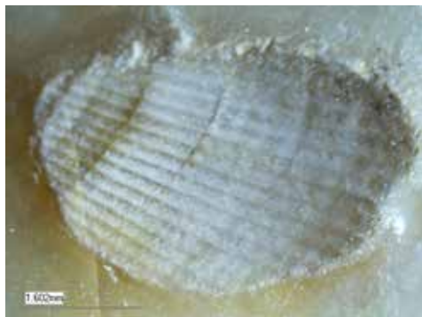
Obr. 2 Schránka mlže. Skutečná velikost je cca 5 mm.
