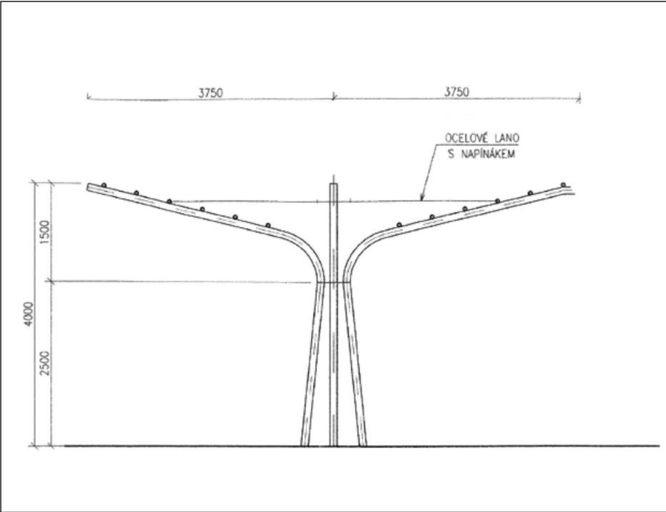
Jednoduchý bokorys podoby prototypu samonosné ocelové konstrukce, která po popnutí rychlerostoucí rostlinou může poskytnout stín na nehostinných stanovištích, jakými jsou například velké parkovací plochy.
