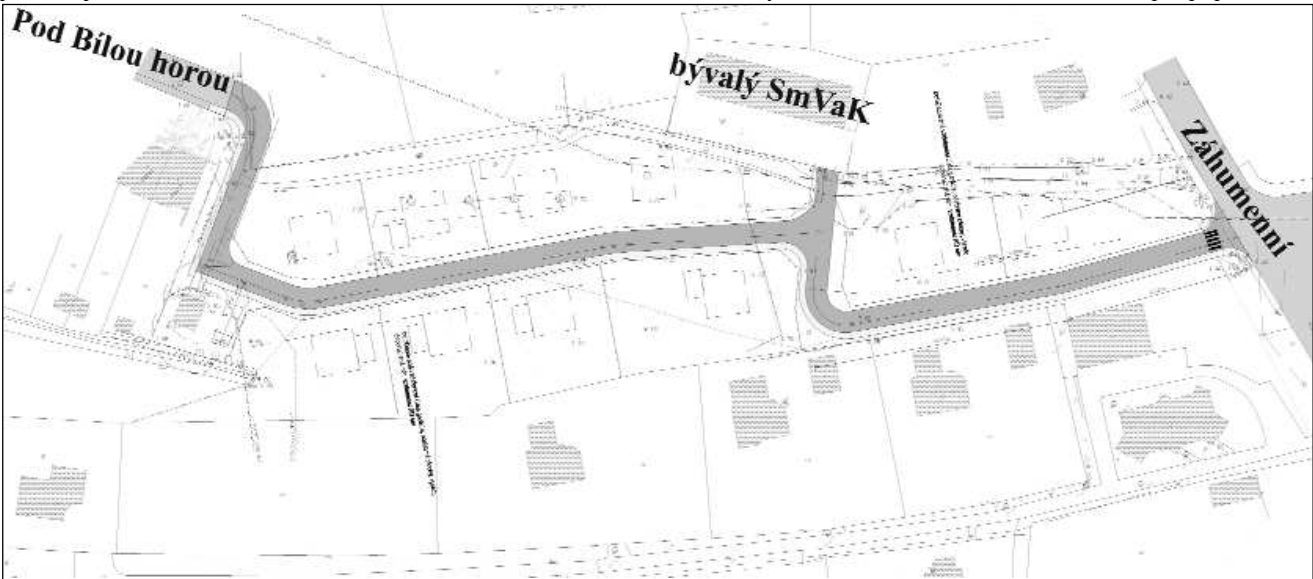
Návrh na propojení komunikací Pod Bílou horou, Husovy ulice a Záhumenní.
