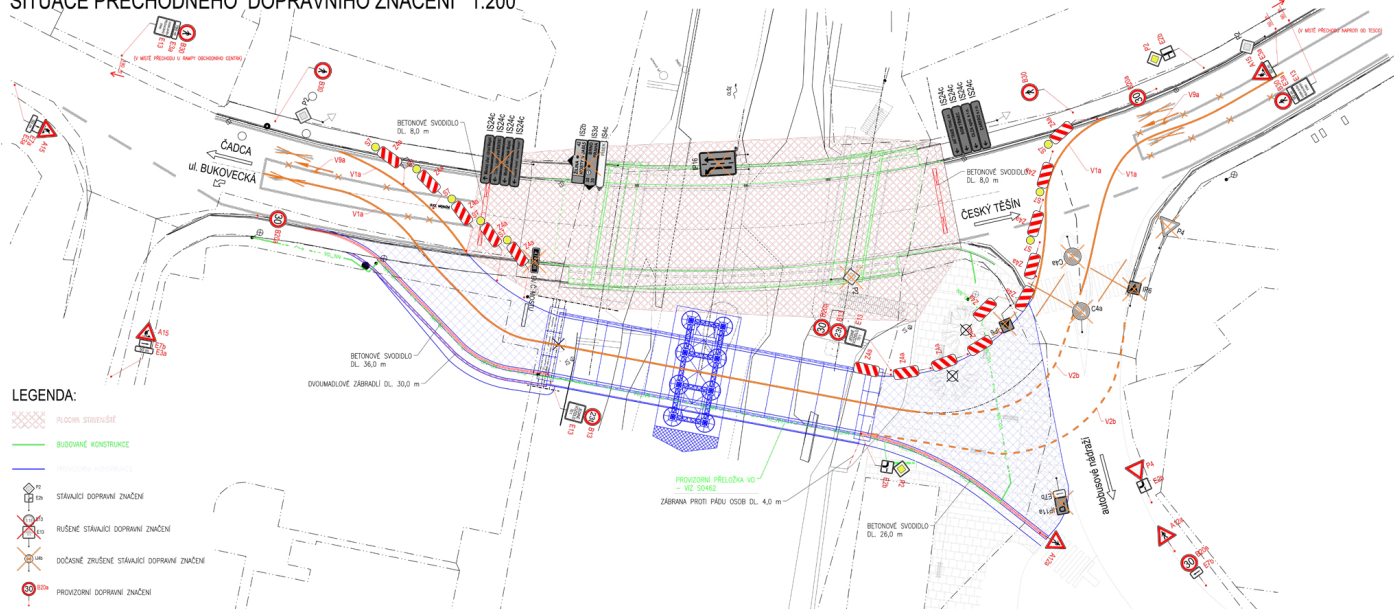
SITUACE PŘECHODNÉHO DOPRAVNÍHO ZNAČENÍ 1:200
