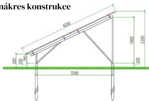
nákres konstrukce
