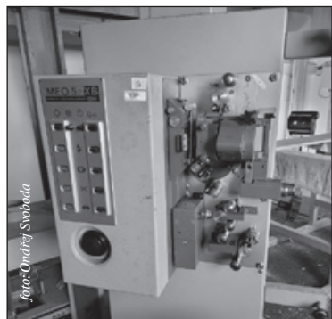
35 mm projektor Meo XB 5, jež dvě funkce jsou instalovány v promítárně
