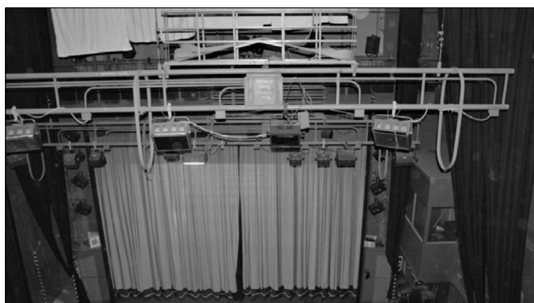
Pohled na horizontální osvětlovací baterii z druhé tzv. vyvažovací lávky
