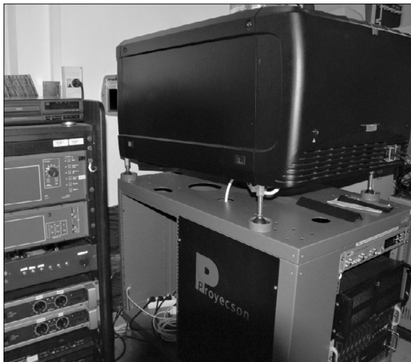
Současná promítací technika. Vpravo nahoře projektor Barco, pod ním ve stojanu rozcestník signálu Gefen, multimediální počítač a náhradní zdroj. Vlevo ve stojanu zvukový procesor Dolby, dekodér digitálního záznamu zvuku Dolby a koncové zesilovače
