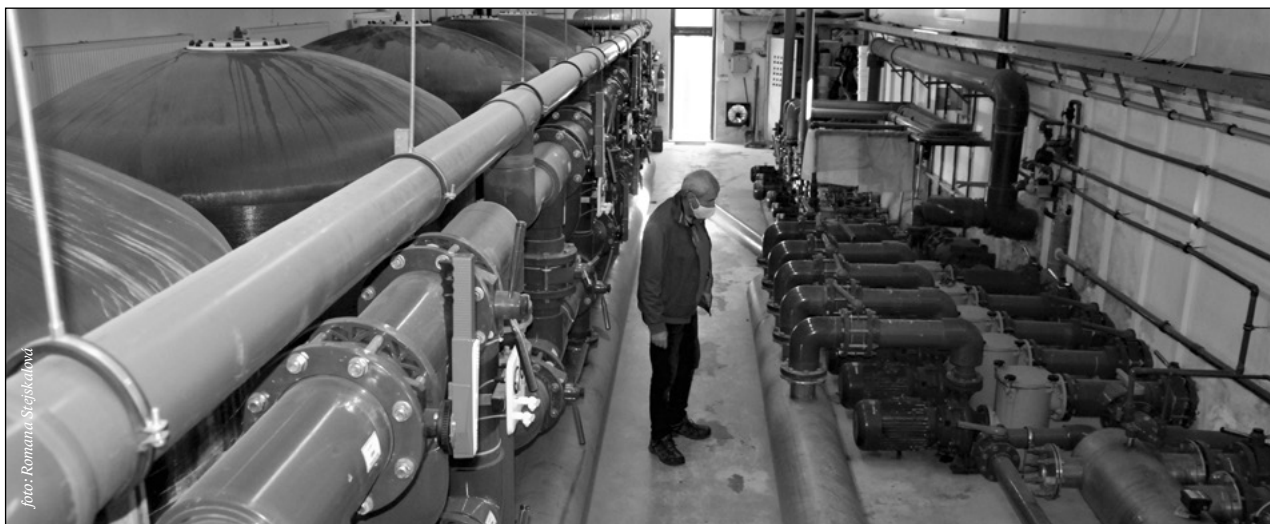
V zadní části strojovny se nachází vpravo cirkulační čerpadla pro atrakce akvaparku. Každá atrakce je vybavena vlastním zařízením (čerpadlo proti proudu, čerpadlo chrlíče)
