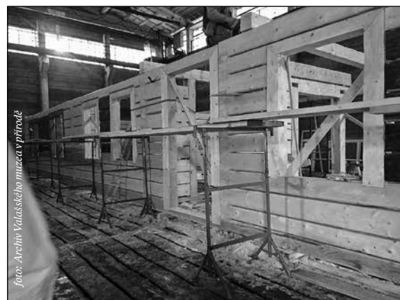
Nový Libušín se začne skládat na místě vyhořelého. Jakmile to počasí dovlí a bude dokončena oprava základu, převevou řemeslníci na Pustevny konstrukci, která se již chystá v hale na Bystřičce
